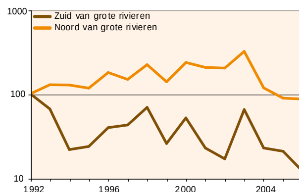
Figuur 2. De waarnemingen uitgesplitst naar regio's.
