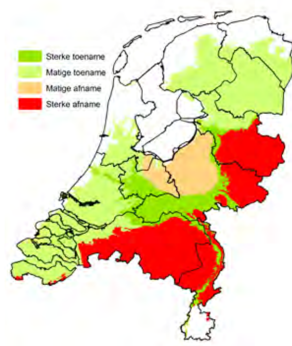
Figuur 3. De trends sinds 1992.
