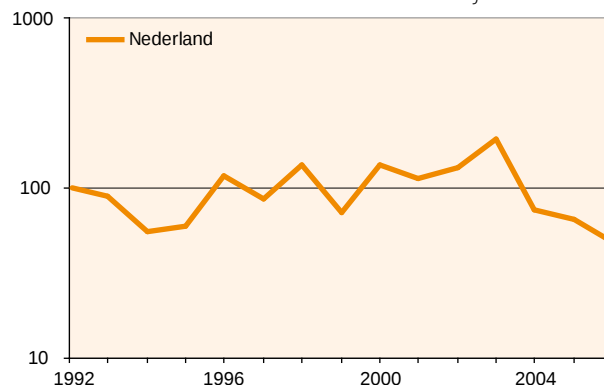
Figuur 1. De landelijke trend van het landkaartje.
