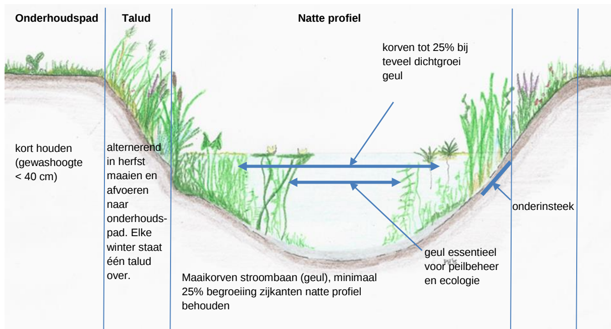
Afbeelding 3: Overzicht dwarsprofiel watergang met onderhoudsconcept (Figuur: Paul Hendriks)
